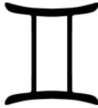
GEMINI2=
